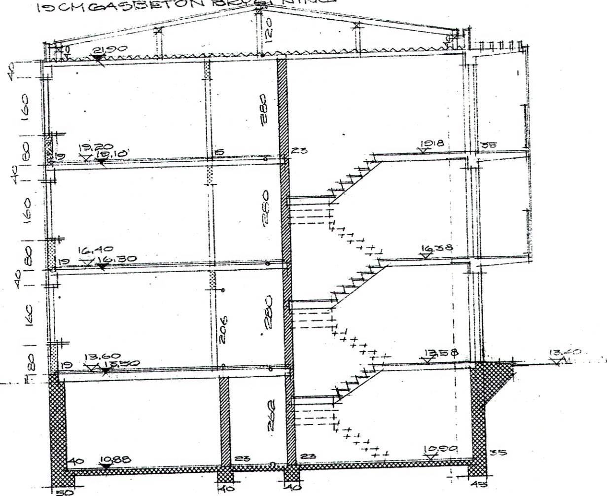
SNIT A-A
